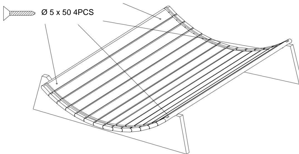
Untere Lamelle
