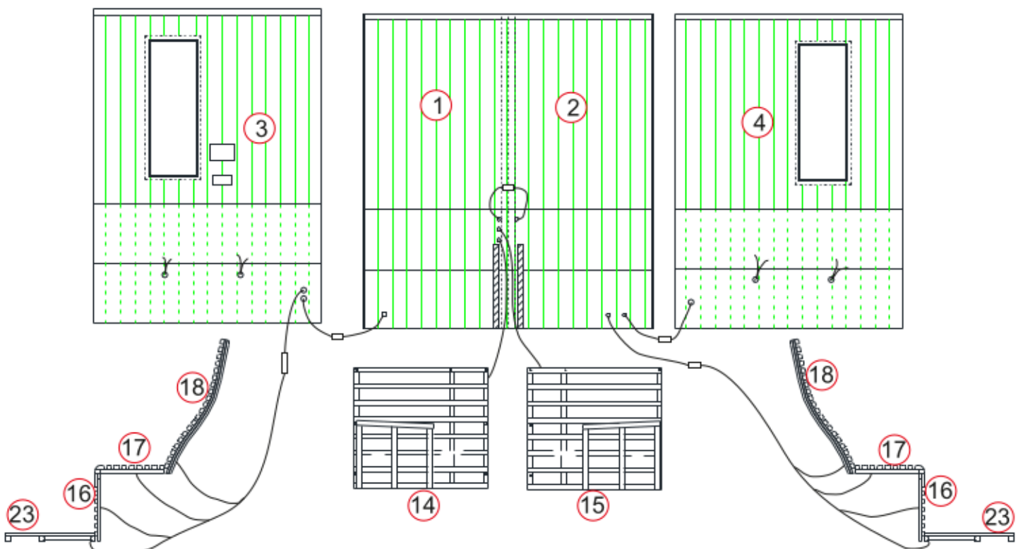
Anschlussplan
