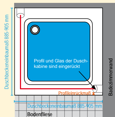
Beispiel: MasterClass Tür mit Seitenwand
